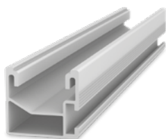
Montageschiene K2 SingleRail 36 Material: Aluminium EN AW-6063 T66
