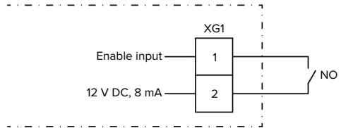
Fig. 15: Schematic circuit diagram: Enable input
