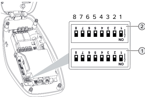
Afb. 12: Dipschakelaar (uitleveringstoestand)
